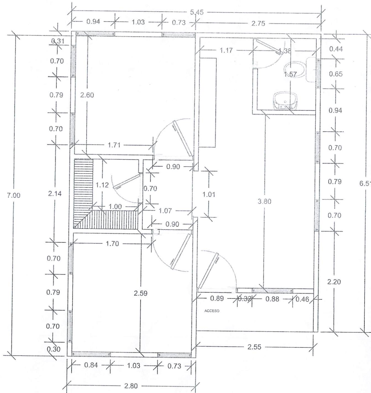
PLANTA DIMENSIONADA DISPENSARIO MEDICO DGDC
